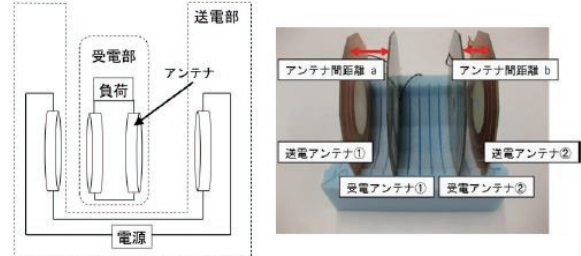
提案のアンテナ配置構造
