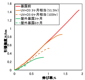
図4. 暴露前後の引張強度
