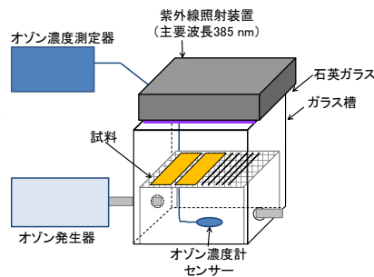
図1. 複合試験装置概略図
