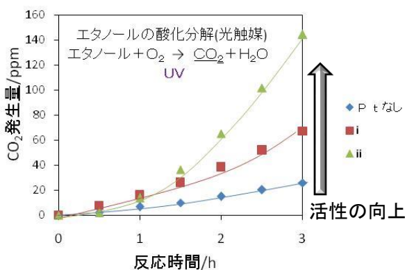
図1. エタノールガス分解活性に対するPt担持方法の影響 i: メタノール/塩化白金酸水溶液中にTiO 2 を導入した多孔質シリカを浸漬して光照射 ii: TiO 2 を導入した多孔質シリカの細孔に塩化白金酸水溶液を注入し、メタノール水溶液中で光照射
